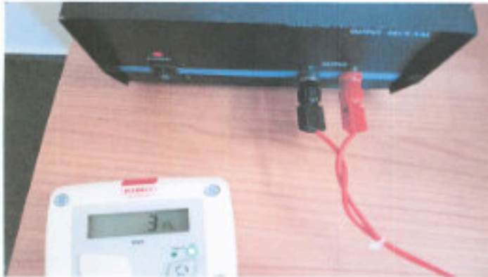
9:48 Uhr Streambox mit Förderleistung von 50m 3 /h Druckdifferenz 3 Pascal (Pa)
