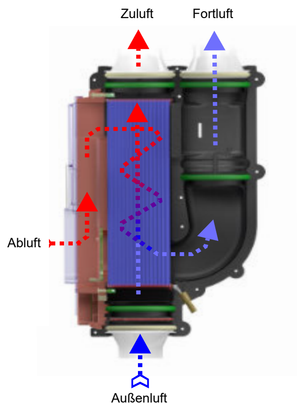
Gehäuseschnitt mit Strömungswegen
